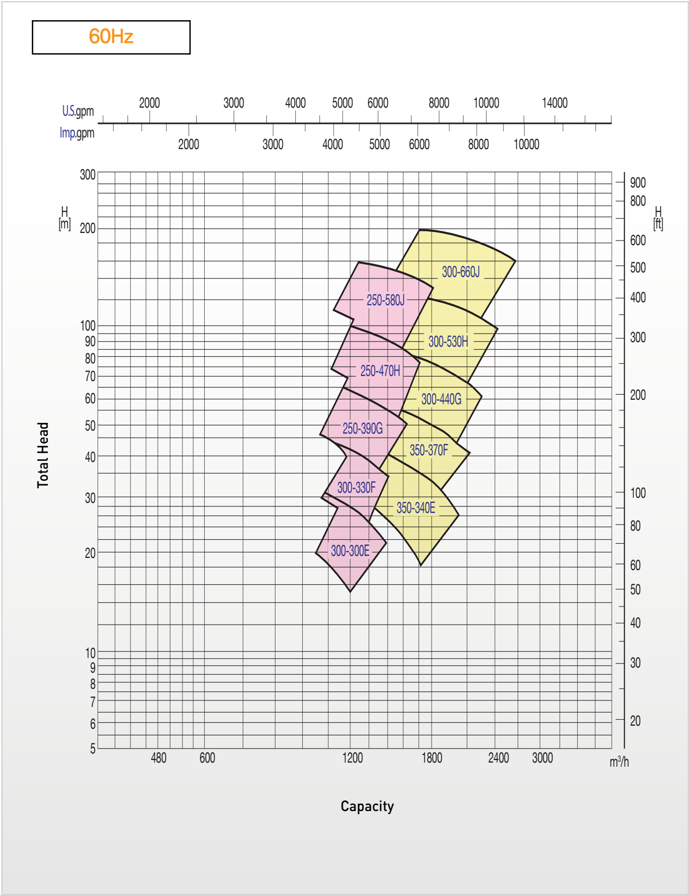
선택도 Selection Chart (Impeller Type : E~J)
